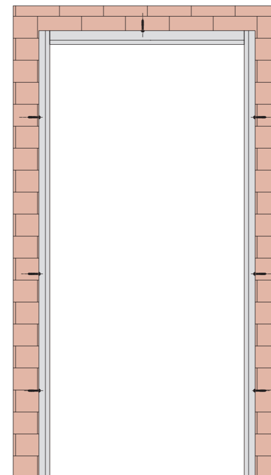
Tradiční montáž do zdiva
