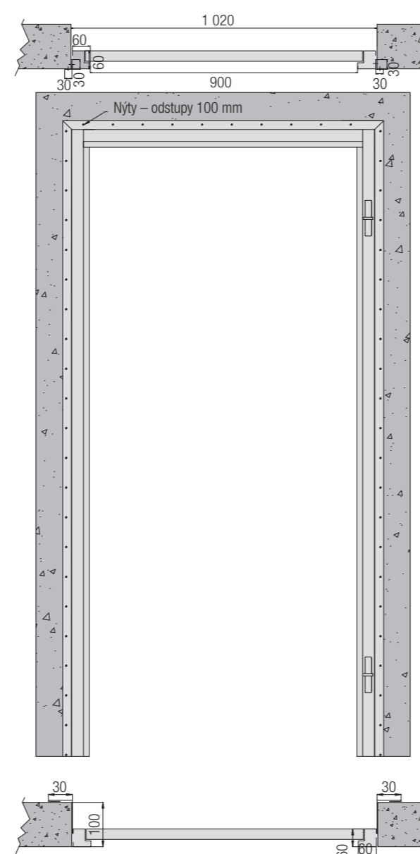
Montáž do stěny z izolačních panelů
